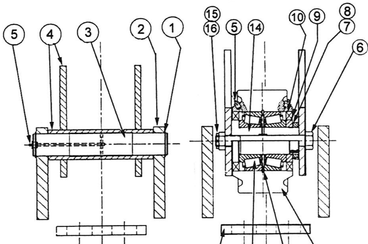
SECCIÓN AA
