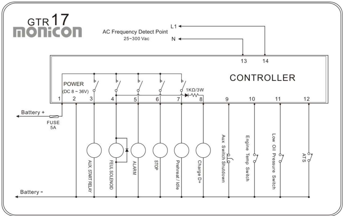
Fig. 5 Controller wiring
