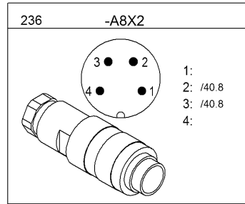
HCM I-Signal
