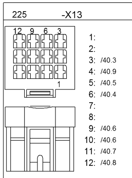
Wire harness HCM
