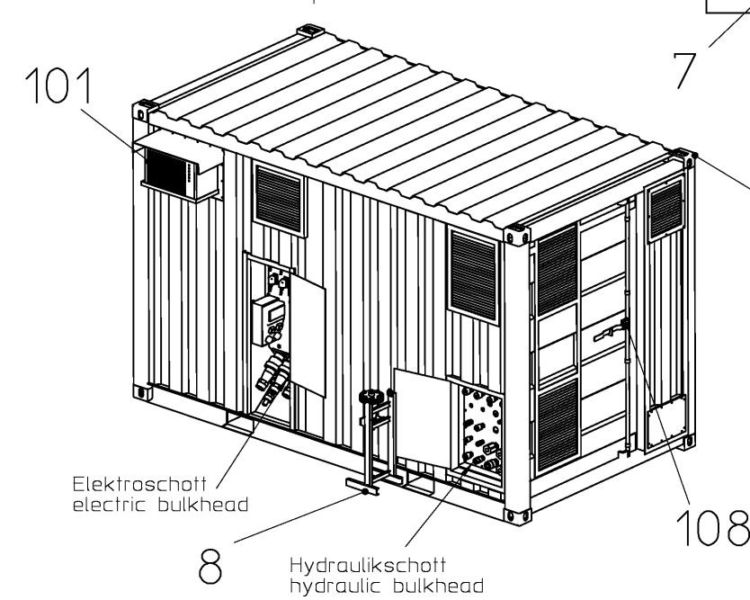
Allg. Ansicht 1 1:60
