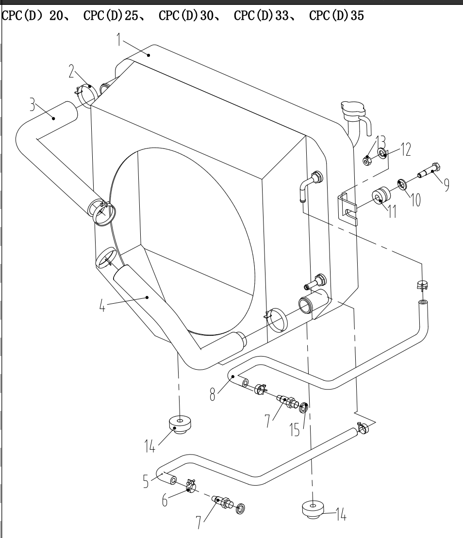
图 09 冷却系统(490/495、4DA1/4DC1、C240PKJ、4JG2) COOLING SYSTEM (490/495、4DA1/4DC1、C240PKJ、4JG2)
