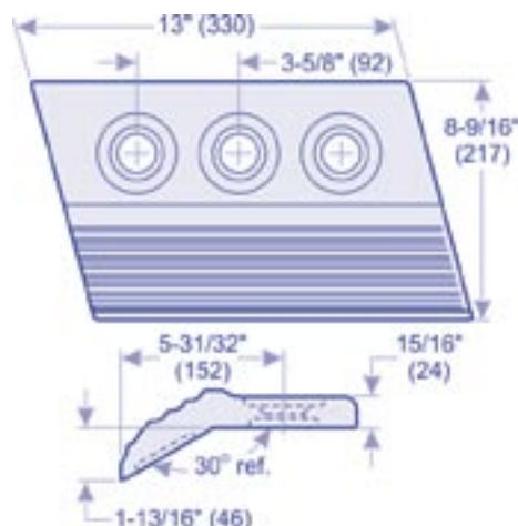
WA600-TCR (WA600) shown WA600-TCL (WA600) opposite
