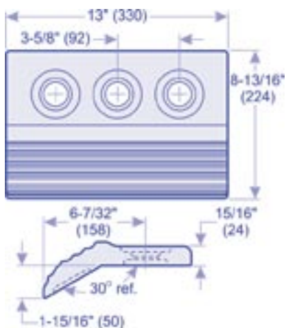
WA600-TCC (WA600)
