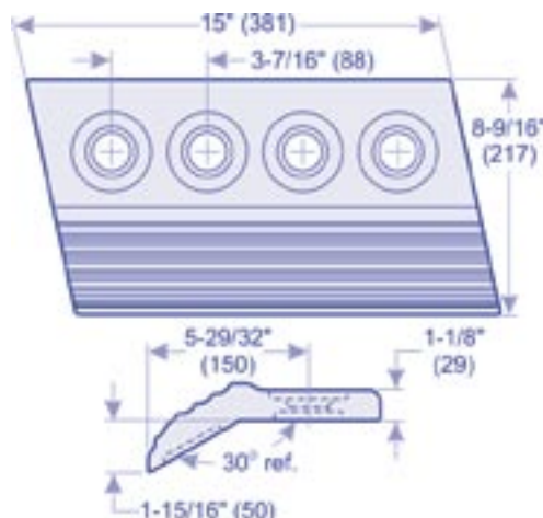
WA700-TCR (WA700) shown WA700-TCL (WA700) opposite
