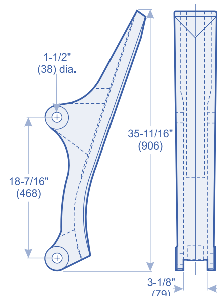
195-78-72410HX 111.0 lbs. (49.9 kgs.)
