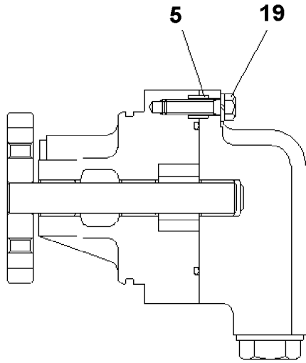
断面 B - B Section B-B
