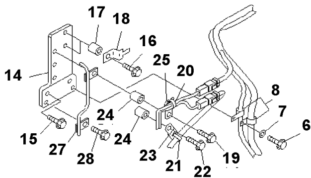
A 詳細 Detail A
