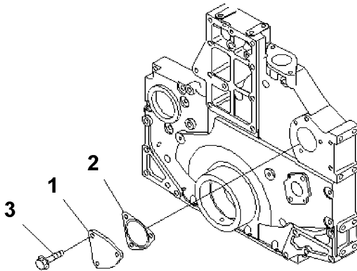
フロントカバー Front Cover
