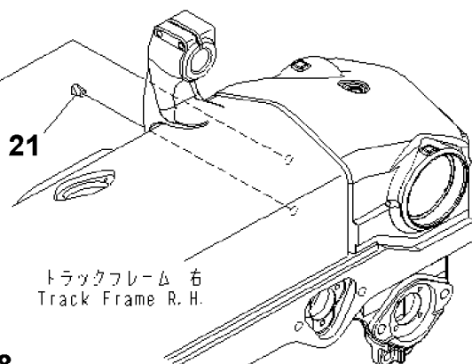
ボギー吊りブラケット Bogie Lifting Bracket
