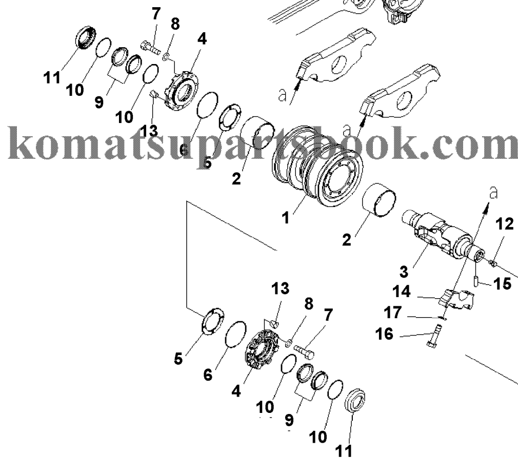
トラックフレーム 右 Track Frame R.H.
