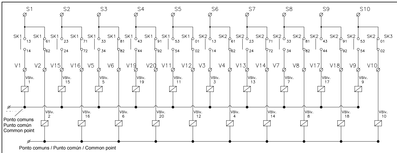
Diagrama de ligação / Diagrama de conexión / Schematic diagram
