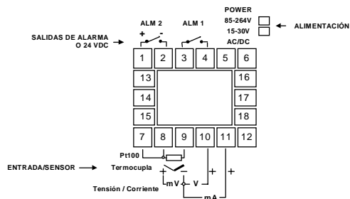
Figura 1 - conexiones eléctricas del indicador
