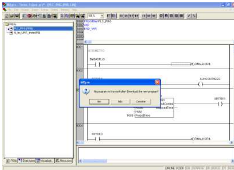
Figura 122 – Confirmação do download para o CLP
