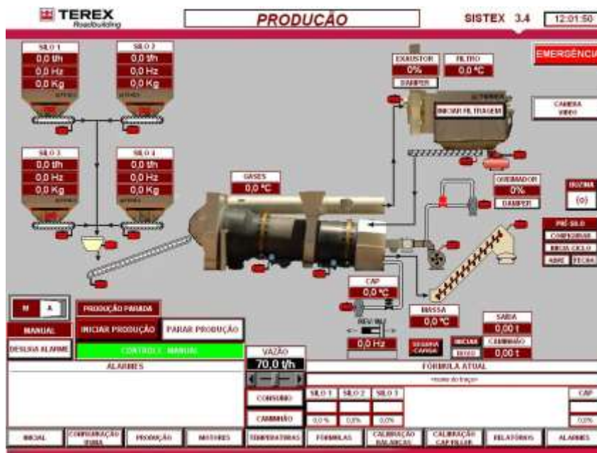
Figura 19 – Acompanhamento de la producción
