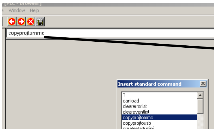
Figura 91 – Fazendo download para a memória do CLP – Cópia da lógica de programação
