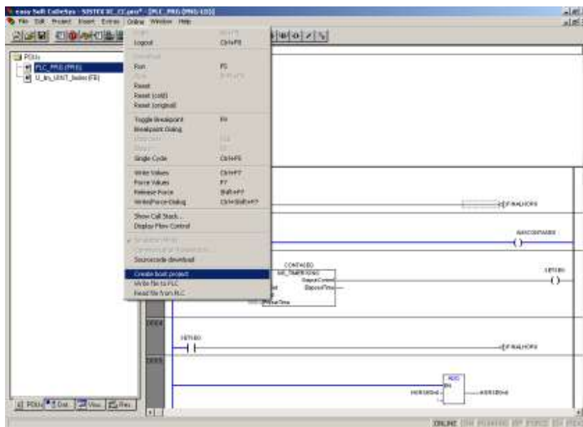
Figura 122 – Conclusión del descarga del CLP
