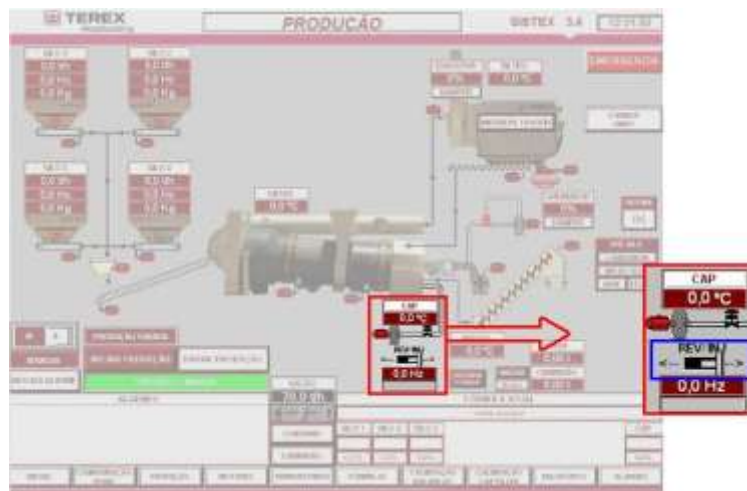
Figura 24 – Acionamento da reversão/injeção da bomba de CAP
