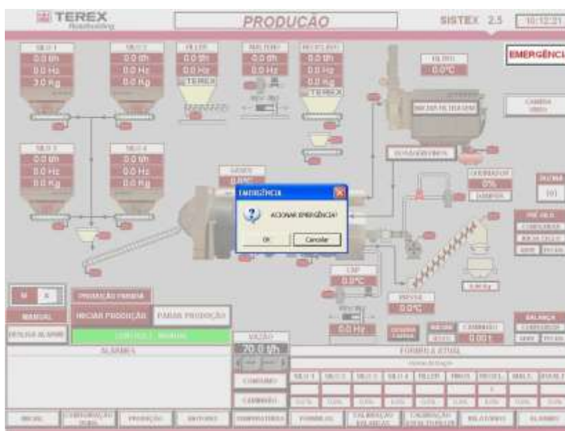
Figura 6 – Accionamiento del botón de EMERGENCIA
