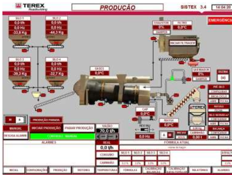
Figura 26 – Acionamentos da Usina de Asfalto
