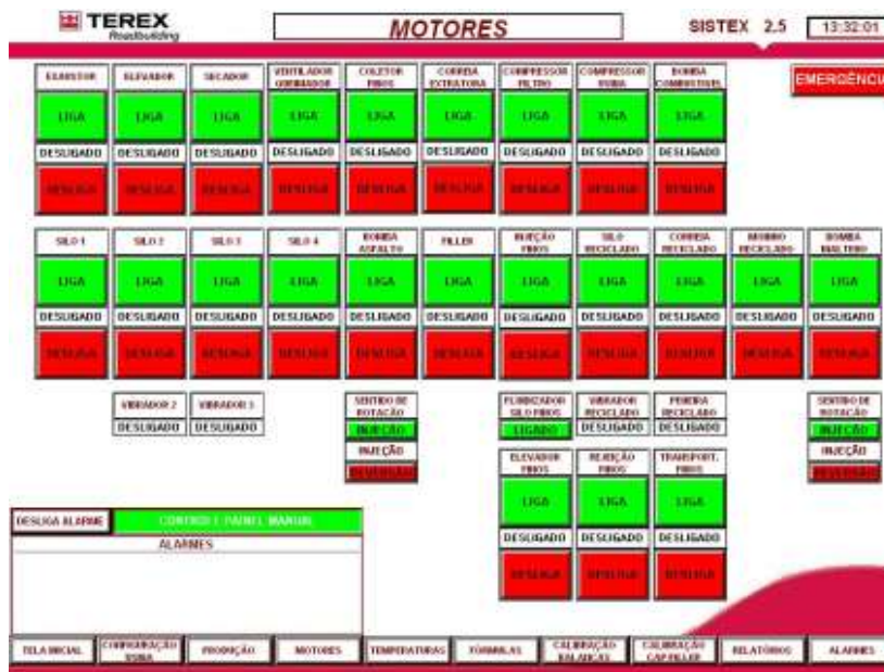
Figura 20 – Acompanhamento através da tela de motores
