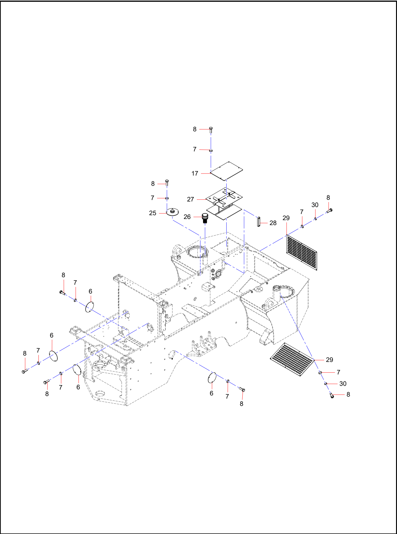
7-4 后车架总成
