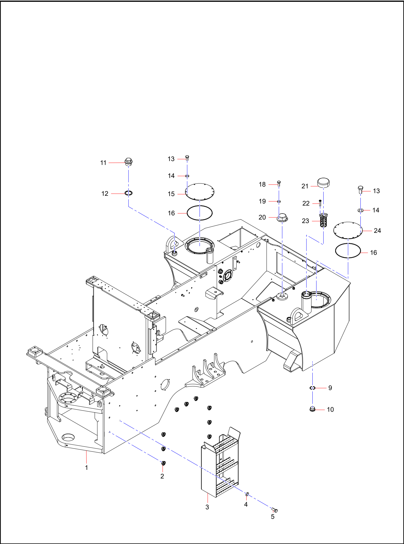
7-2 后车架总成
